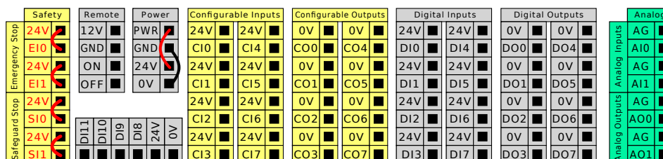
Skupiny vstupů a výstupů (I/O).
