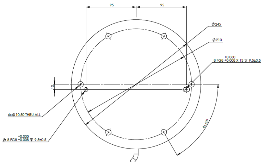
1.1: Pohled na základnu robota zespodu
